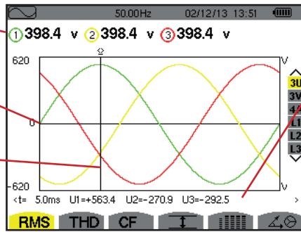
Abbildung 53: Bildschirm zur RMS-Anzeige bei 3U
