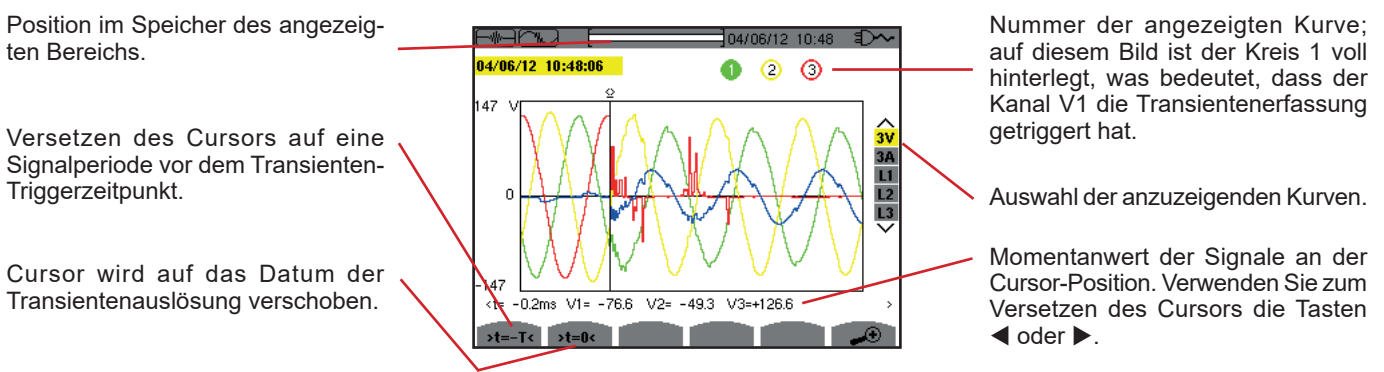
Abbildung 40: Beispiel für die Anzeige von Transienten in Form von Kurven bei der Anschlussart Dreiphasig 4 Leiter
