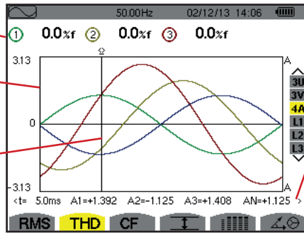
Abbildung 59: Bildschirm zur THD-Anzeige bei 4A
