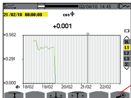
Abbildung 95: cos φ (L1) abgeschlossener Lade-/Berechnungsvorgang ohne MIN-AVG-MAX für eine dreiphasige Quelle mit Neutralleiter
