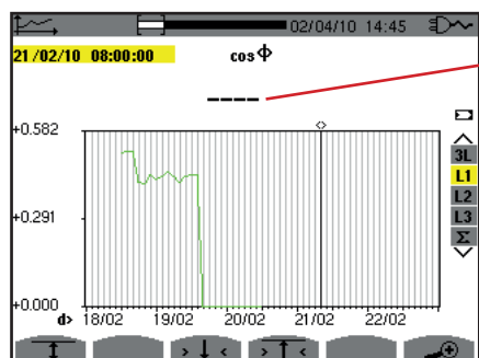
Abbildung 94: cos φ (L1) frühzeitiges Ende des Lade-/Berechnungsvorgangs..
