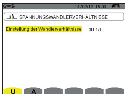
Abbildung 27: Bildschirm Spannungsverhältnisse im Menü Stromwandler und Übersetzungsverhältnisse – Fall einer Anordnung ohne Neutraleiter
