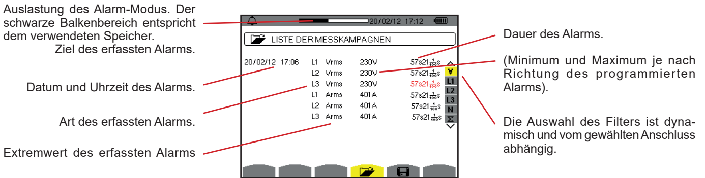
Abbildung 75: Bildschirm Alarm-Liste
