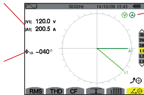
Abbildung 72: Bildschirm zur Anzeige des Zeigerdiagramms bei L1
