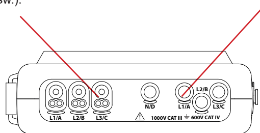
Abbildung 4: Anschlussbuchsen
