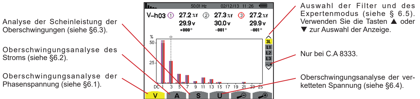
Abbildung 41: Bildschirm des Modus Oberschwingungen
