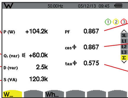
Abbildung 103: Bildschirm zur Anzeige der Leistungen und abgeleiteten Gesamtgrößen bei Σ
