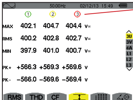
Abbildung 63: Bildschirm zur Anzeige von Max-Min bei 3U
