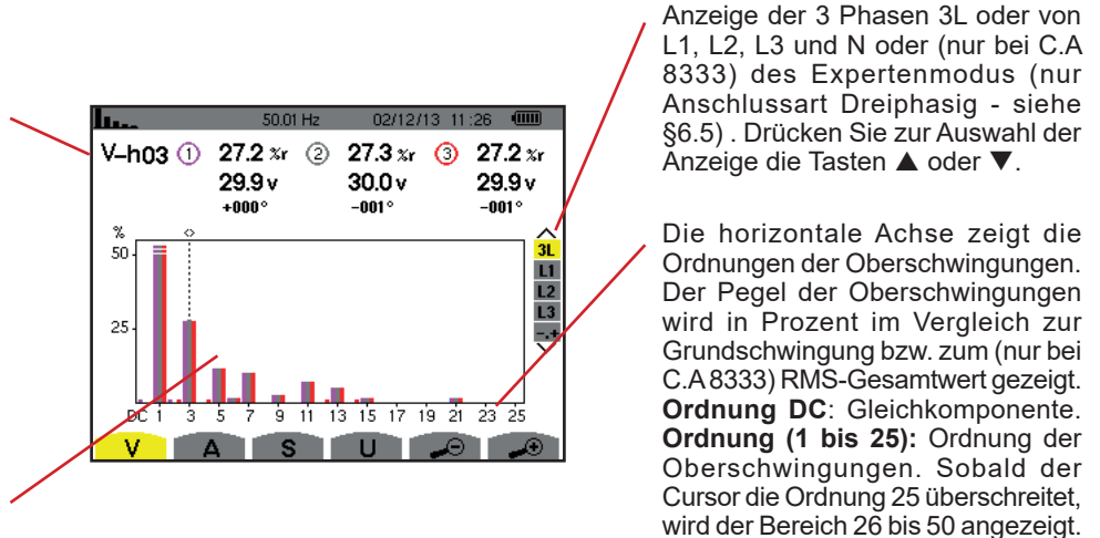
Abbildung 42: Anzeigebeispiel für Oberschwingungen der Phasenspannung bei 3L
